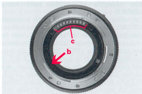
Came R (b) et contacts électriques (c)
